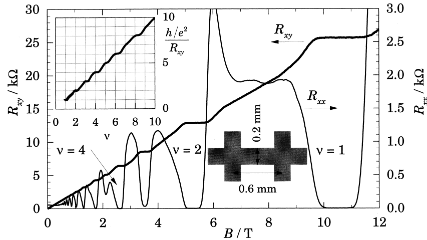
Obrázok 4.2: Meranie kvantového Hallovho javu, prevzaté z John H. Davies, 1998. Označenia R_{xx} a R_{xy} na obrázku zodpovedajú našim R_L a R_H .
