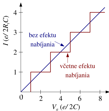
Obrázok 6.9: Ideálna teoretická I-V charakteristika v režime coulombovskej blokády pre C_1 = C_2 = C a R_t = R_{t1} \gg R_{t2} .
