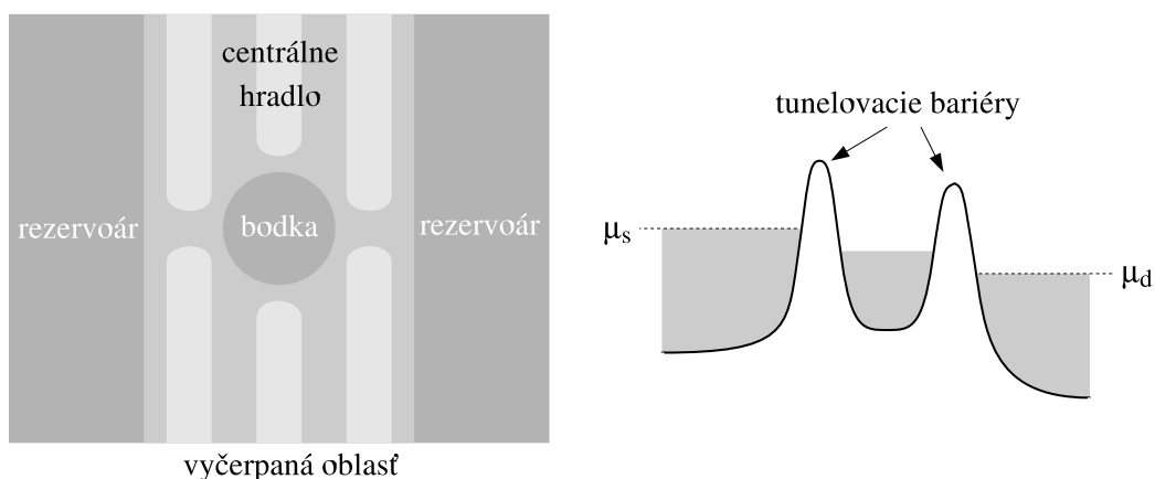
Obrázok 6.11: Planárna štruktúra pre jedoelektrónové tunelovanie a coulombovskú blokádu. Štruktúra funguje ako jedoelektrónový tranzistor, pretože potenciál ostrovčeka je možné riadiť napätím na centrálnom hradle.
