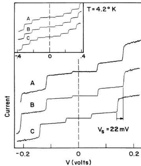
Obrázok 6.10: Experimentálne zmerané (A) a vypočítané (B, C) coulombovské schodište pre 10–nanometrovú kvapku In v dielektrickej matici. Jednou elektródou je vodivý substrát, druhou je hrot STM mikroskopu. (Wilkins et al., 1989)
