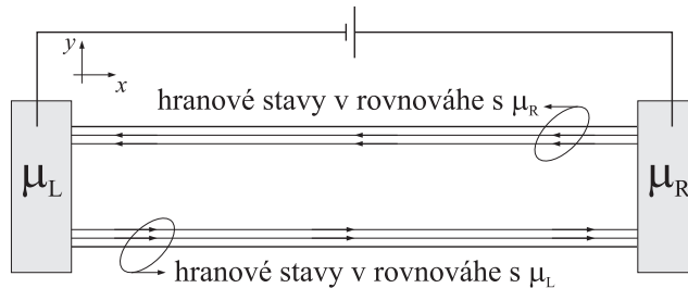
Obrázok 4.11: Kvantový Hallov jav v dvojterminálovej vzorke.
