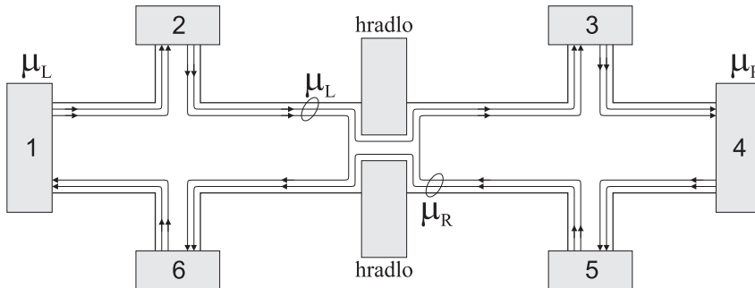
Obrázok 4.14: Hallov kríž s dvojítm hradlom.
