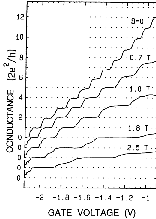
Obrázok 2.5: Kvantovanie balistickej vodivosti v magnetickom poli, merané VanWeesom.
