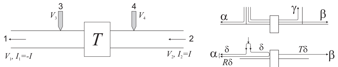
Obrázok 3.7: Štvortermínálový systém.
