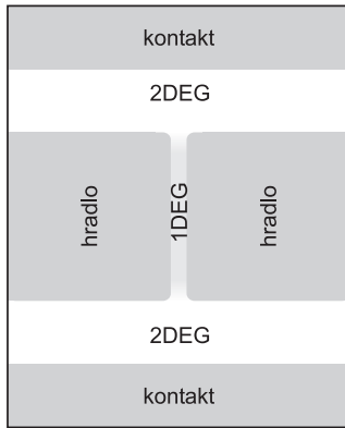
Obrázok 2.3: Meranie vodivosti, B. van Wees et. al. , Phys. Rev. Lett. 1988.
