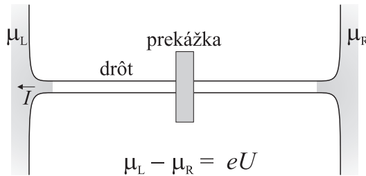
Obrázok 3.1: Mezoskopický vodič s prekážkou. Vodivosť G = I/U je tzv. dvojterminálová vodivosť, pretože sa meria potenciálový rozdiel U medzi prúdovými terminálmi L a R .
