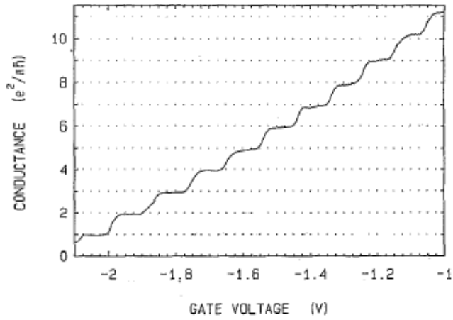
Obrázok 2.3: Meranie vodivosti, B. van Wees et. al. , Phys. Rev. Lett. 1988.
