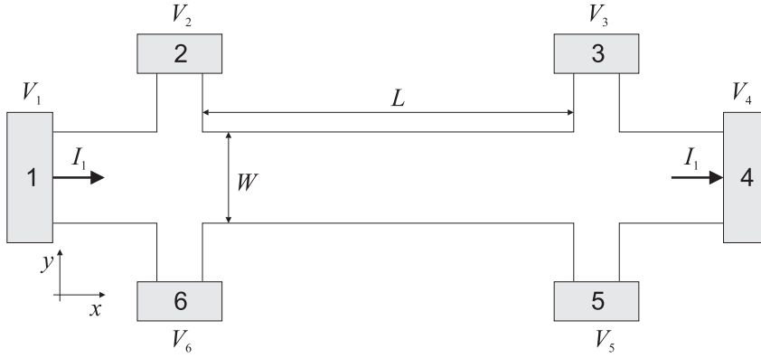
Obrázok 4.1: Typická geometria vzorky pre meranie kvantového Hallovhov javu.
