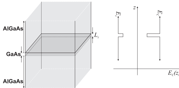
Obrázok 1.1: Pribeh dna vodivostného ( E_C ) a vrcholu valenčného pásu ( E_V ) v tenkej vrstve GaAs zovretej dvomi polonekonečnými AlGaAs vrstvami. Vrstva GaAs je pre vodivostné elektróny potenciálovou jamou, pre \text{Al}_x\text{Ga}_{1-x}\text{As} s x \approx 0.3 je asi 0.3 eV hlboká.
