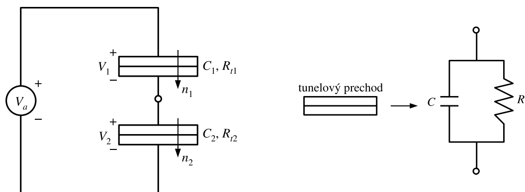
Obrázok 6.6: Náhradný obvod pre dvojbariérovú štruktúru z obrázku 6.2. Kovový “ostrovček” je spojený s kladnou a zápornou elektródou cez dva slabé tunelové spoje modelované ako doskové kondenzátory s kapacitami C_1 a C_2 . R_t sú odpory tunelových spojov a n_1 resp. n_2 označuje počet elektrónov, ktoré na ostrovček pretunelovali cez spoj 1 resp. 2.
