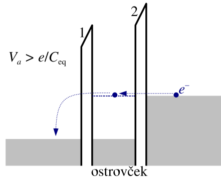
Obrázok 6.8: Ostrovček pod napätím. Napätie > e/C_{eq} umožňuje tunelovanie.
