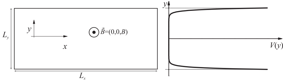
Obrázok 4.3: Potenciál definujúci okraje vzorky (schématicky).
