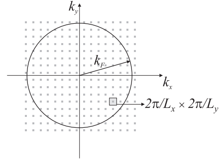
Obrázok 1.4: Znáznorenie 2D stavov v k -priestore.
