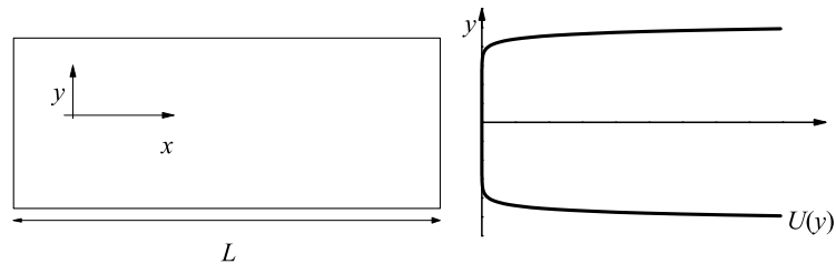
Obrázok 1.5: Schematické znázornenie priebehu väzobného potenciálu na hranách 2D vzorky konečnej šírky.
