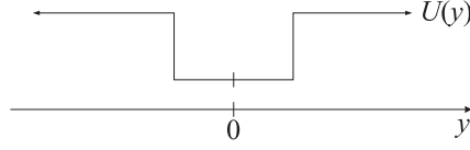
Obrázok 1.6: Vázobný potenciál ako pravouhlá jama.
