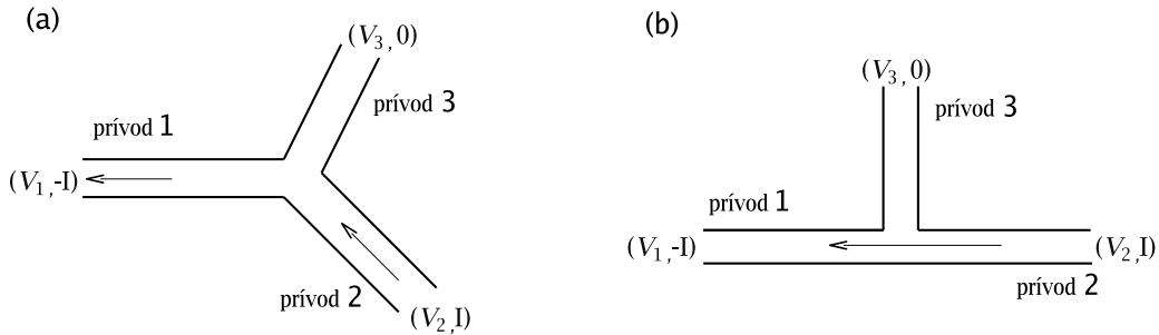
Obrázok 3.6: (a) Trojterminálový systém s dvomi prúdovými terminálmi a napäťovou sondou 3. (b) To isté pre rovný balistický vodič
