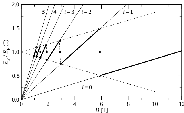
Obrázok 4.10: Fermiho hladina elektrónového 2D plynu v magnetickom poli B .
