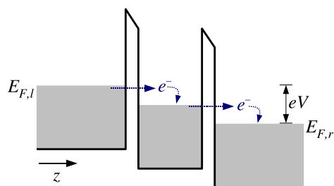
Obrázok 6.2: Tunelovacia dvojbariéra. Predpokladáme sekvenčné tunelovanie, ktoré sa realizuje, ak je vzdialenosť medzi bariérami väčšia ako stredná voľná dráha medzi dvomi zrážkami.
