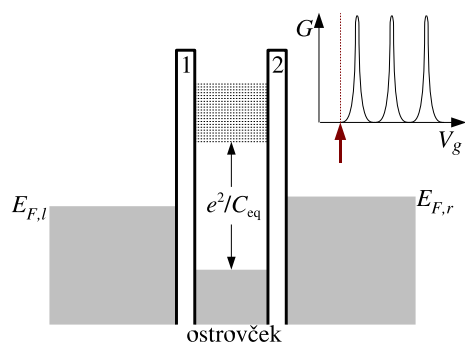
Obrázok 6.14: Píky konduktancie a energetický diagram dvojbariérovej štruktúry pre V_g mimo rezonanciu.
