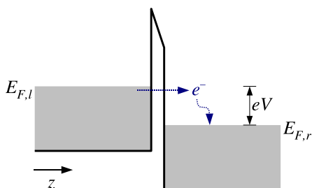
Obrázok 6.1: Tunelovacia bariéra kov - dielektrikum - kov pod napätím.
