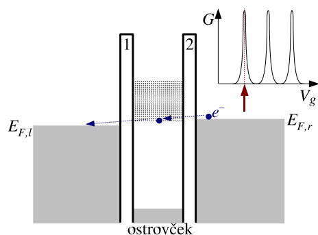
Obrázok 6.15: Píky konduktancie a energetický diagram dvojbariérovej štruktúry pre V_g v rezonancii.
