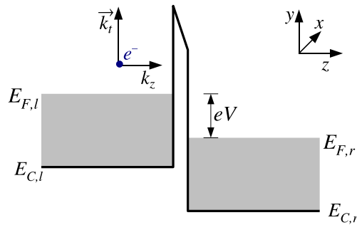
Obrázok 6.3: Model tunelovacej dvojbariéry v systéme kov - dielektrikum - kov.
