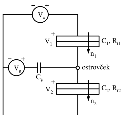
Obrázok 6.12: Náhradná schéma pre jedoelektrónový tranzistor.
