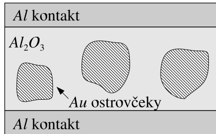
Obrázok 6.4: Prierez štruktúrou so zlatými zrníčkami zaliatymi v dielektriku Al_2O_3 .
