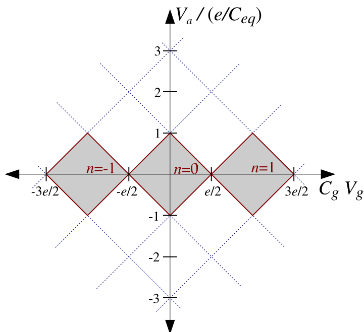
Obrázok 6.13: Diagram stability pre jedoelektrónový tranzistor v prípade C_g = C_2 = C , C_1 = 2C . Tmavé oblasti zodpovedajú hodnotám V_a a V_g , pre ktoré je tunelovanie na ostrovček zakázané pri rôznych hodnotách n . Oblasti teda reprezentujú stabilné režimy pre rôzne celočíselné počty elektrónov na ostrovčeku. Mimo týchto oblastí jedoelektrónové tunelovanie funguje štandardným spôsobom.
