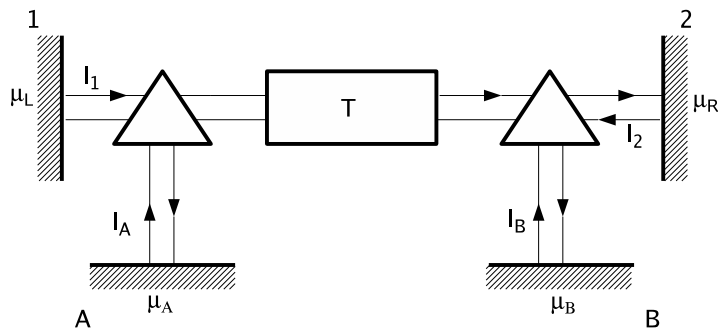
Obrázok 3.9: Meranie potenciálu vo vodiči s prekážkou ideálnymi potenciometrami
