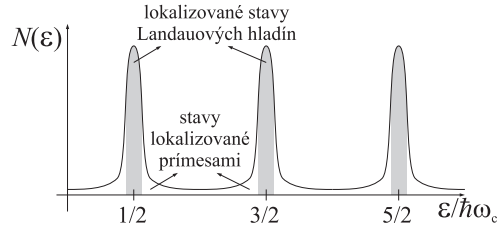
Obrázok 4.8: Vďaka prímiesnym stavom je N(E) nenulové aj mimo Landauových hladín. Preto môže Fermiho energia s meniacim sa B spojite prechádzať cez lokalizované stavy medzi Landauovými hladinami.
