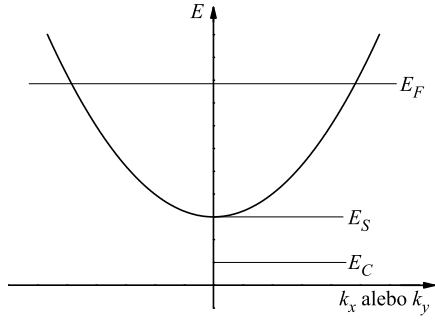
Obrázok 1.3: Disperzný zákon 2D elektrónov (vzťah (1.11) pre n = 1 ).
