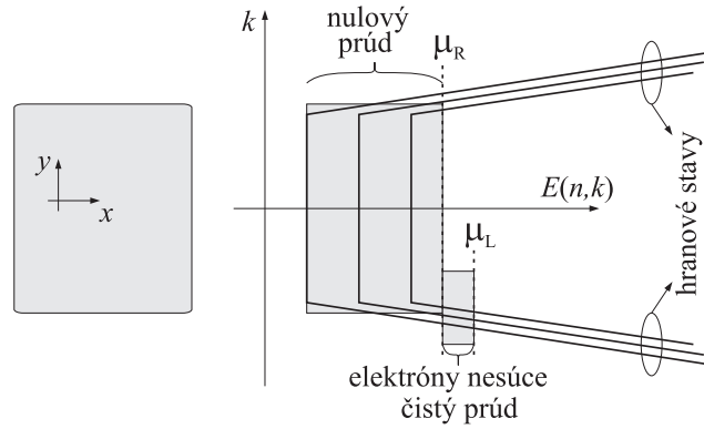
Obrázok 4.12: V stavoch s energiou menšou ako Fermiho energia sa prúdy od stavov k_x presne kompenzujú prúdmi stavov -k_x . Čistý prúd nesú len elektróny, ktoré sú injektované z ľavého kontaktu do hranových stavov idúcich zľava do prava s energiou v intervale [\mu_L, \mu_R] .
