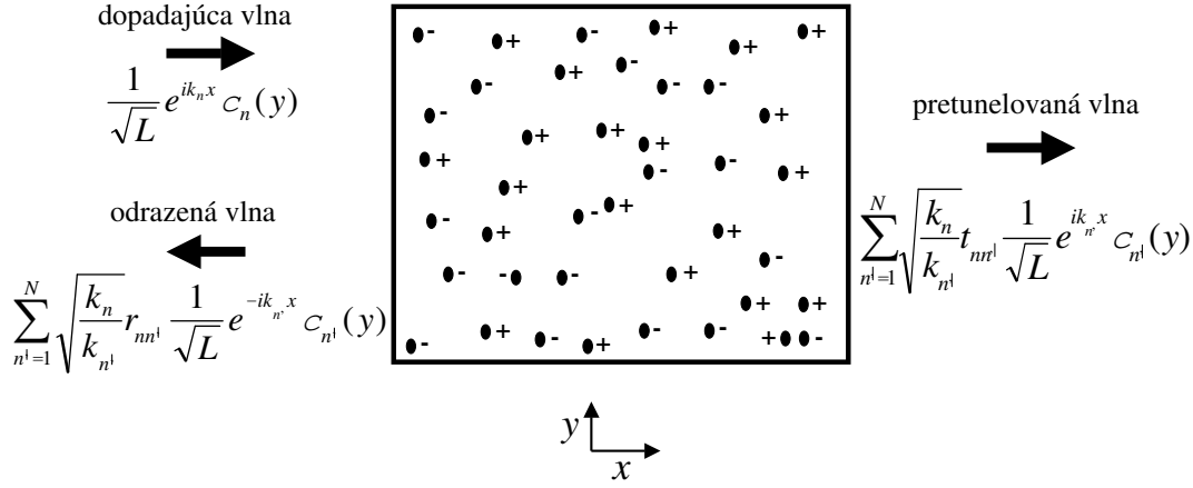
Obrázok 3.2: Mezoskopický vodič s náhodne rozloženými prímiesami. Prímiesi so znamienkom plus/mínus sú príť a žlivé/odpudivé. Vytvárajú náhodný potenciál U_I(x, y) , ktorý dopadajúcu vlnu čiastočne odráža a čiastočne prepúšťa (pozri text).
