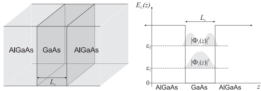
Obrázok 1.2: Znázornenie potenciálu viažúceho vodivostné elektróny v tenkej (2D) GaAs vrstve zovretej dvoma polonekonečnými AlGaAs vrstvami. Dno vodivostného pásu v GaAs, E_C , je tu nulovou hladinou energie (pozri tiež obr. 1.1).
