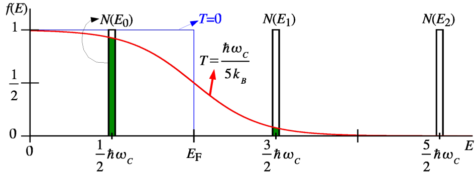
Obrázok 4.9: Fermiho funkcia f(E) pre dve rôzne teploty T v prípade \nu = 1 . V tomto prípade je pri T = 0\text{K} úplne obsadená hladina E_0 = \frac{1}{2}\hbar\omega_c a vyššie hladiny sú úplne neobsadené. Pri malom zvýšení teploty ( k_B T \ll \hbar\omega_c ) umožní Fermiho distribúcia veľmi malé obsadenie hladiny E_1 = \frac{3}{2}\hbar\omega_c . Pritom musí platiť, že f(\frac{1}{2}\hbar\omega_c) + f(\frac{3}{2}\hbar\omega_c) = 1 , odkiaľ po dosadení Fermiho funkcie hneď dostaneme E_F = \hbar\omega_c . Výsledok platí exaktne pre T \rightarrow 0 . Hustoty stavov N(E) sú kvôli jednoduchosti znázornené ako úzke obdĺžniky, v skutočnosti to majú byť \delta funkcie.
