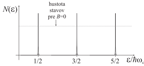
Obrázok 4.7: Hustota stavov N(\varepsilon) vo vzorke bez prímiesí. Keďže medzi dvomi Landauovými hladinami nie sú žiadne stavy, Fermiho hladina sa môže nachádzať jedine na najvyššej obsadenej Landauovej hladine alebo výnimočne presne v strede medzi najvyššou úplne obsadenou a prvou úplne voľnou Landauovou hladinou.
