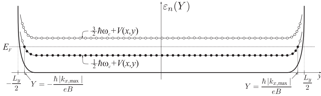
Obrázok 4.4: Landauove hladiny \varepsilon_n(Y) vo vzorke ohraničenej hranovým potenciálom V(y) , ukázaným plnou čiarou. V objeme vzorky je potenciál V(x, y) konštantný (za predpokladu, že absentujú prímesty), takže elektrónové stavy v objeme sú nepohyblivé. Pohybujú sa len elektróny v stavoch v blízkosti hrán, kde má hranový potenciál V(y) nenulový gradient.
