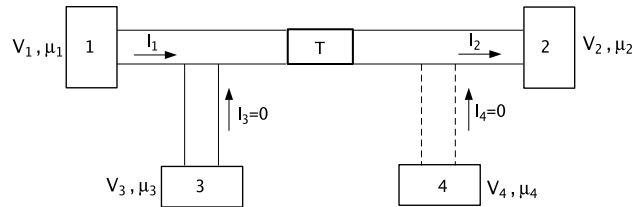
Obrázok 3.10: Štvorbodové meranie potenciálu v jednonábovom vodiči s transmisíou T . Prívody k potenciometrom 3 a 4 sú tiež jednonábové, rovnakého prierezu a z rovnakého materiálu ako je vodič. Predpokladáme, že potenciometre 3 a 4 sú slaboinvázívne. Vtedy výsledný potenciál potenciometra 3 nie je ovplyvnený prítomnosťou potenciometra 4, a naopak. Dôkaz tohto tvrdenia necháme na čitateľa a v texte sa obmedzíme na predpoklad, že keď meria potenciometer 3 tak nie je pripojený potenciometer 4, a naopak.
