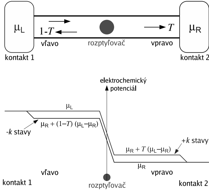
Obrázok 3.8: (a) 1D vodič s jedným rozptyľovačom s transmišiou T . (b) Zmena elektrochemického potenciálu, ukázaná separátne pre elektróny s pozitívnym a negatívnym k .
