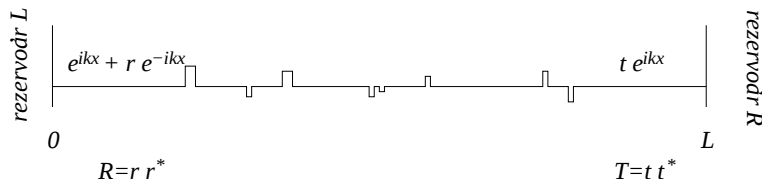
Obrázok 5.1: Jednokanálový vodič dĺžky L obsahuje disorder náhodne rozložených prekážok. Tieto vytvárajú náhodný 1D potenciál zložený z bariér a jám. Z rezervoáru L ide vlna e^{ikx} ( k \equiv k_F ), ktorá sa čiastočne odráža naspäť (s pravdepodobnosťou R ) a čiastočne prechádza cez disorder (s pravdepodobnosťou T ) až do rezervoáru R .
