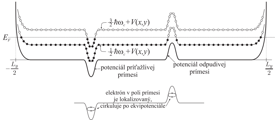
Obrázok 4.5: Schématické znázornenie priestorovej separácie vlnových funkcií s kladným a záporným znamienkom vlnového vektora k_x . Obrázok je nakreslený pre prípad z predchádzajúceho obrázku, keď je obsadená len najnižšia Landauova hladina.
